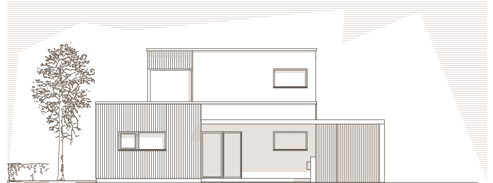
STRASSENANSICHT
